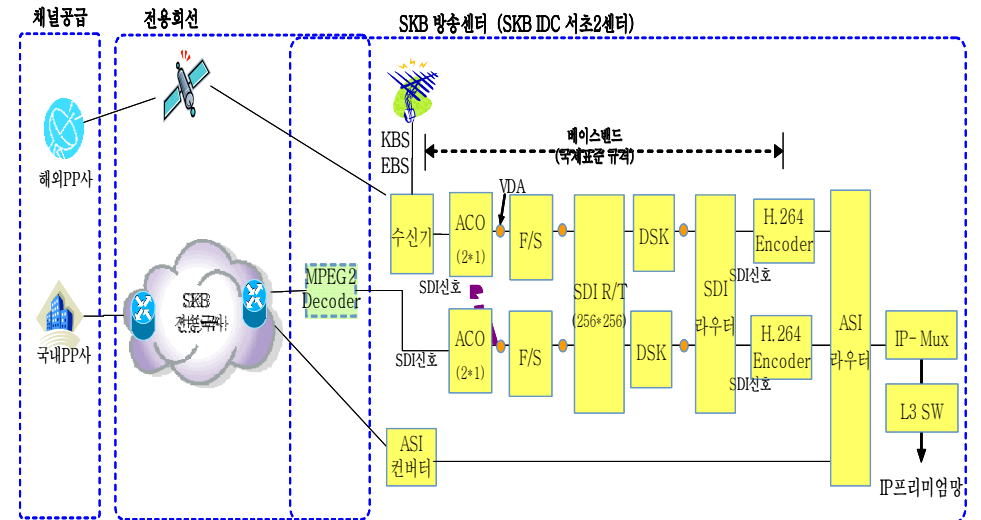
< 피십인의 방송신호 전달 흐름도 >
